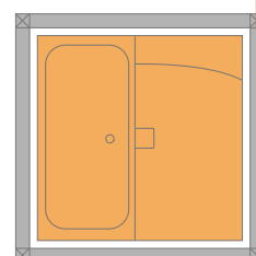
B1717サイズ 浴室寸法1650mm×1650mm (1坪)
